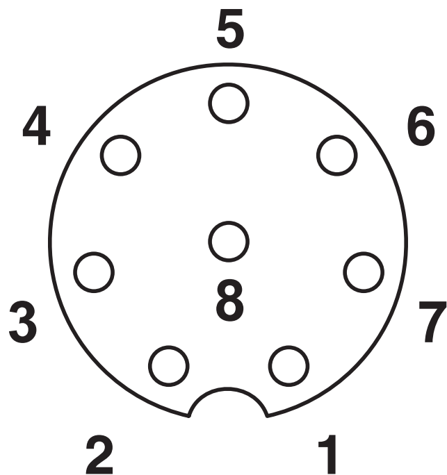
Schematisk ritning
