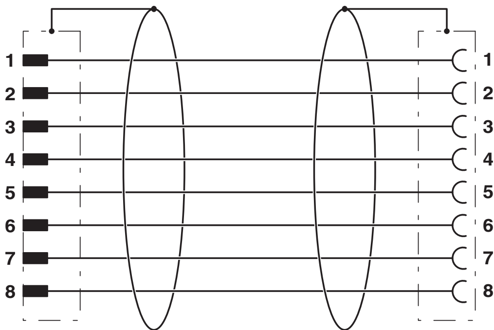
Kopplingsschema
