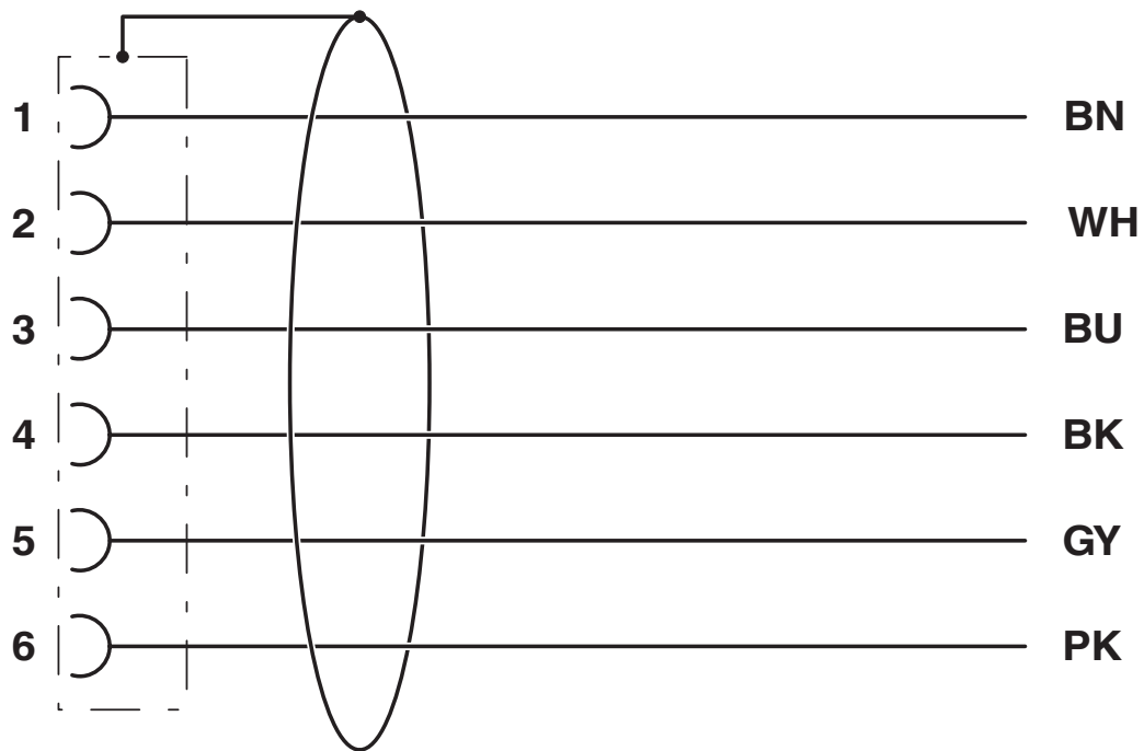
Kopplingsschema
