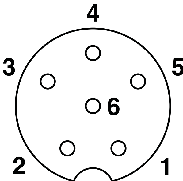
Schematisk ritning
