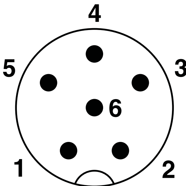
Schematisk ritning
