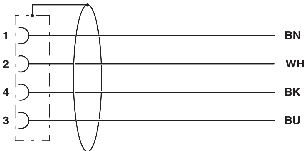
Anslutna M8-honkontakter
