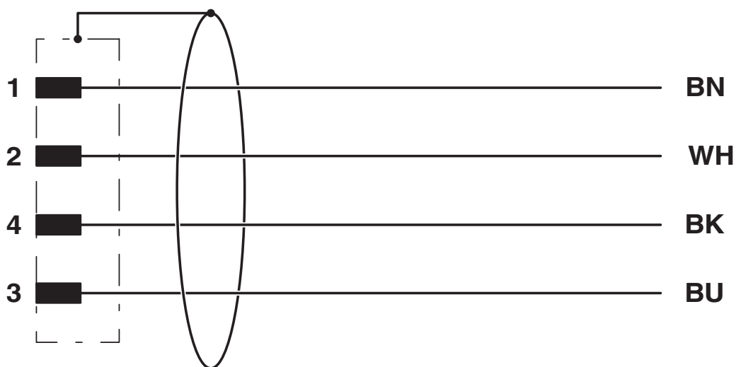
Anslutna M8-han-/honkontakter
