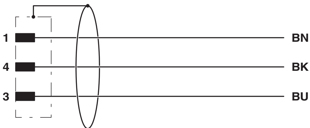
Kopplingsschema
