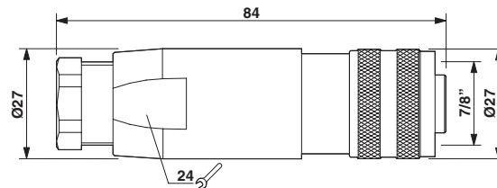
Måttskiss
