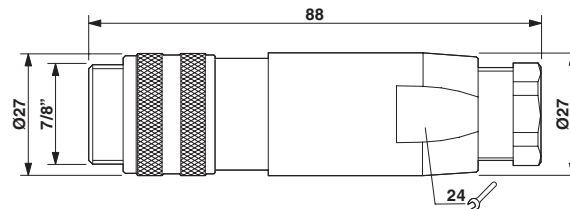
Måttskiss
