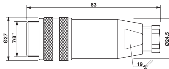
Måttskiss
