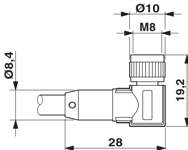
Måttskiss
