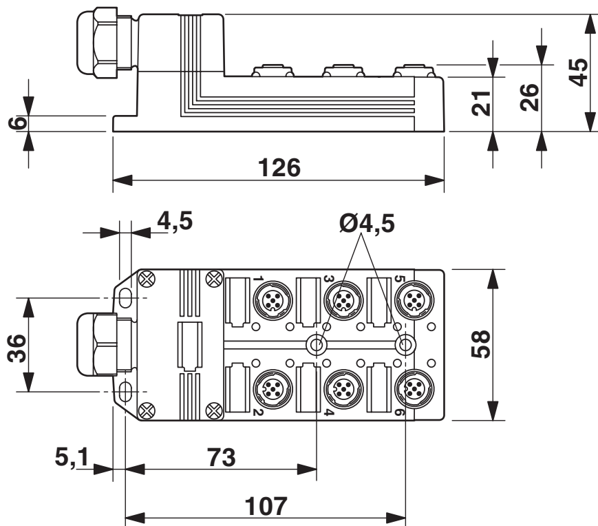
Måttskiss
