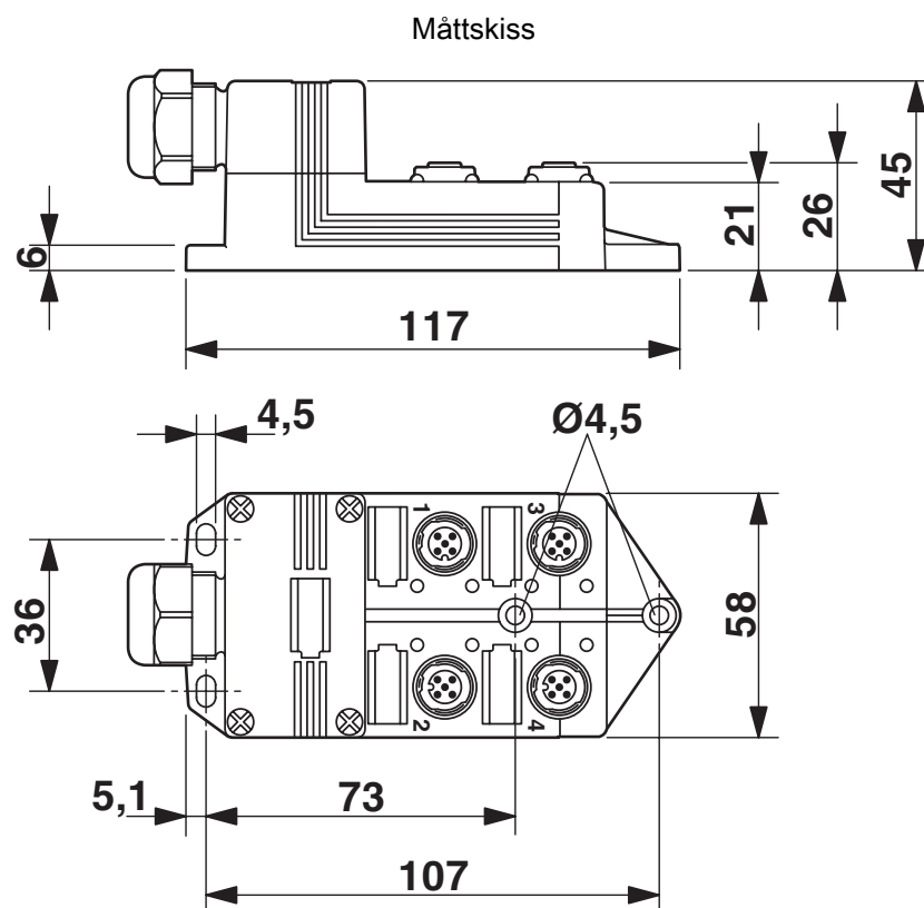
Schematisk ritning
