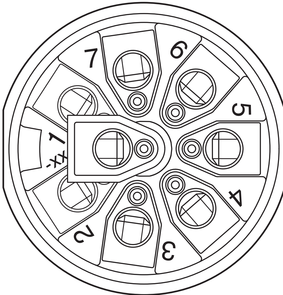
Kabelanslutningssida M12 (skruvanslutning)
