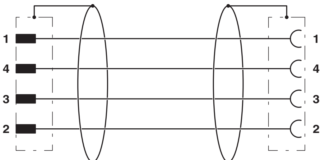
Kopplingsschema
