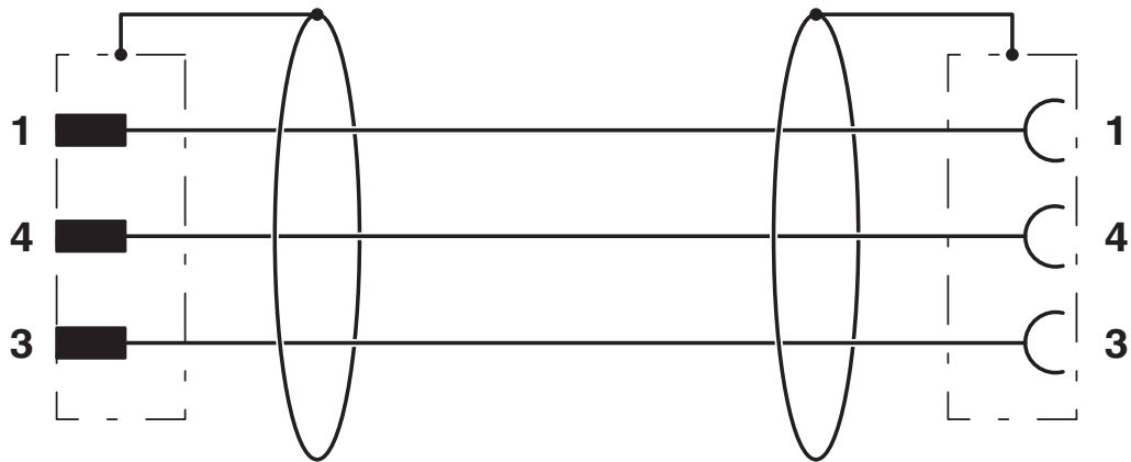
Kopplingsschema
