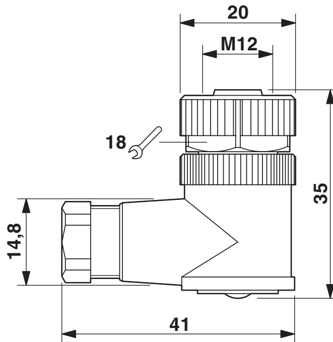
Måttskiss
