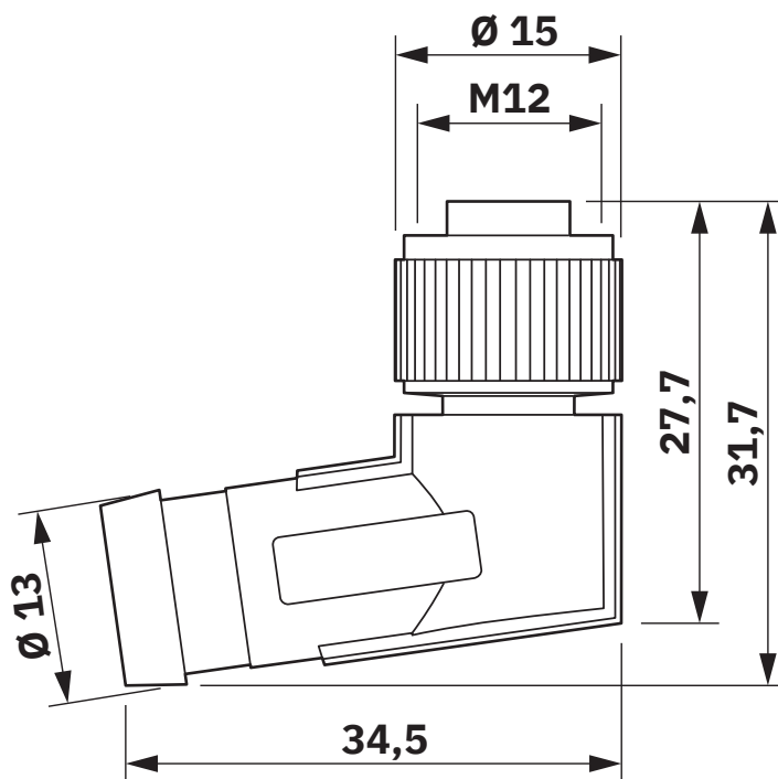
Måttskiss
