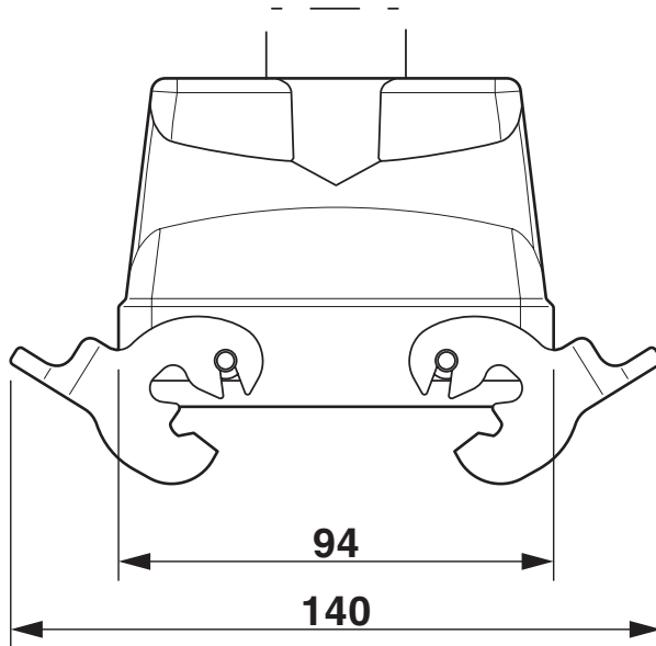
Måttskiss
