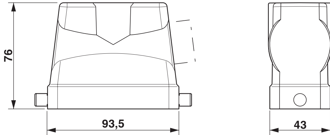
Måttskiss
