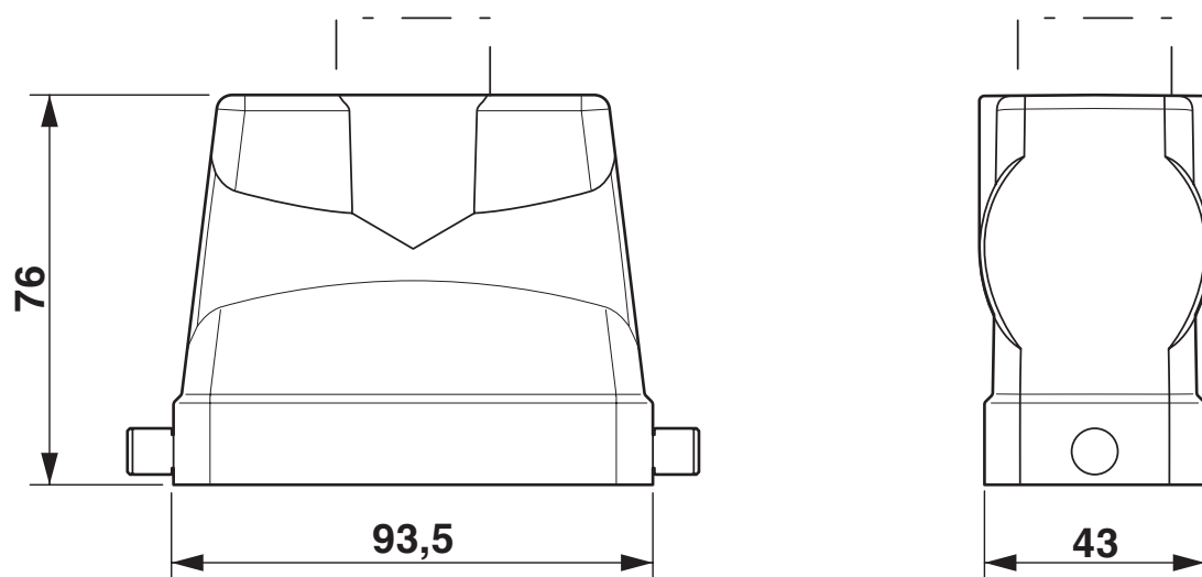
Måttskiss
