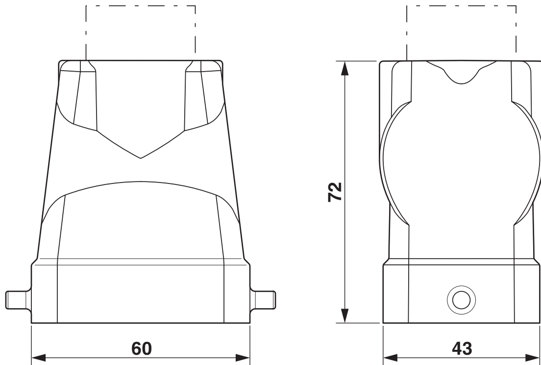
Måttskiss
