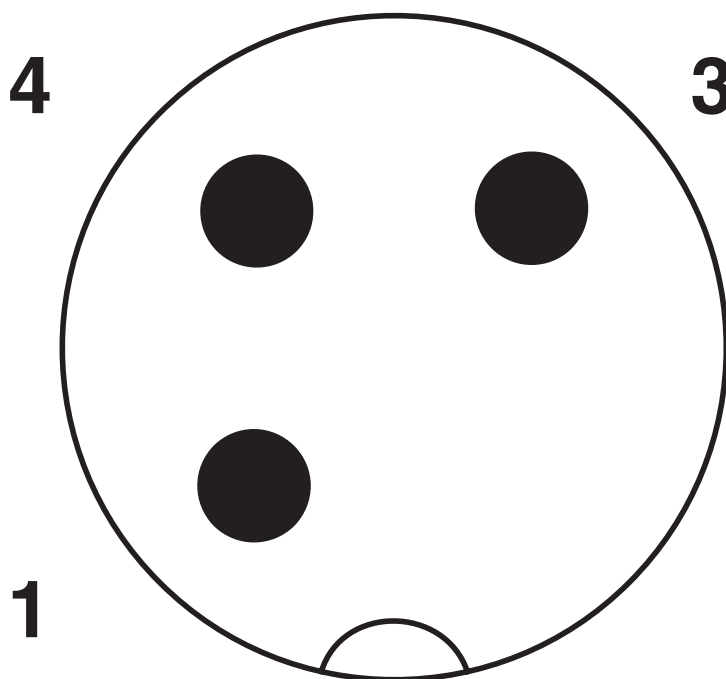
Polbild hane M12, 3-polig, A-kodad, sett från hansidan
