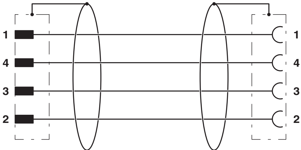
Kopplingsschema
