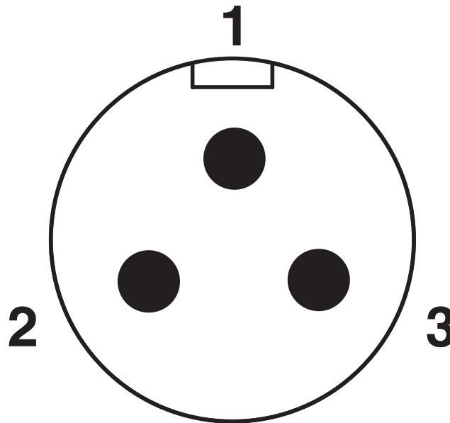
Schematisk ritning
