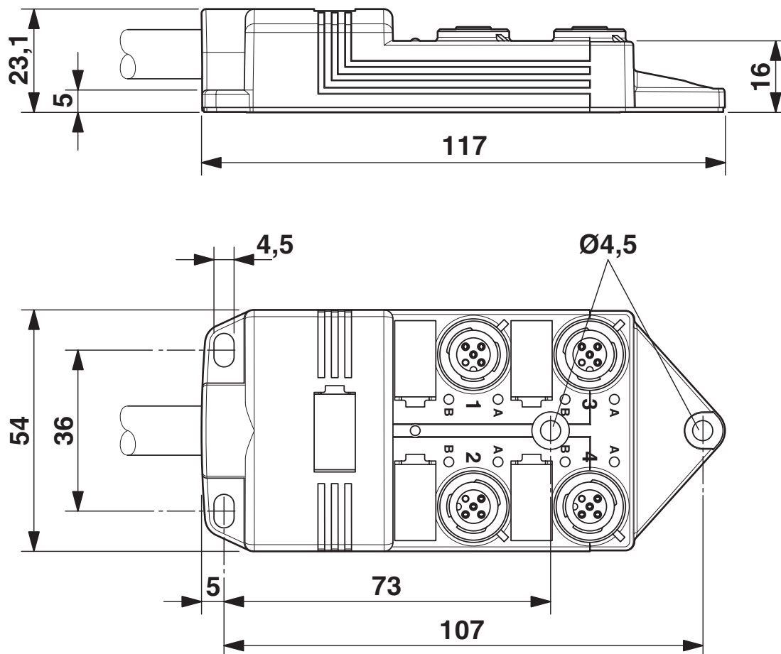
Måttskiss
