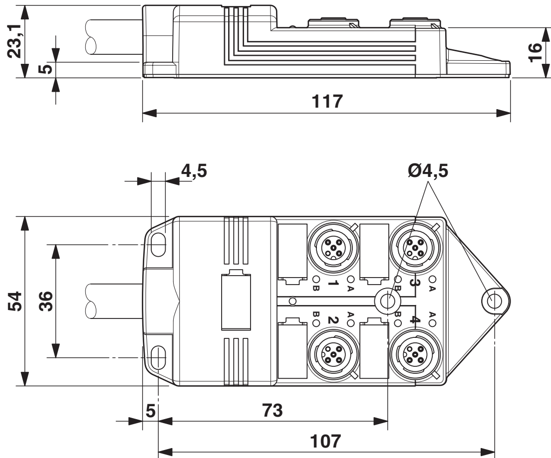
Måttskiss
