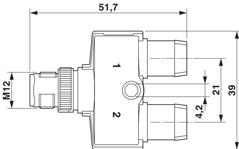
Måttskiss
