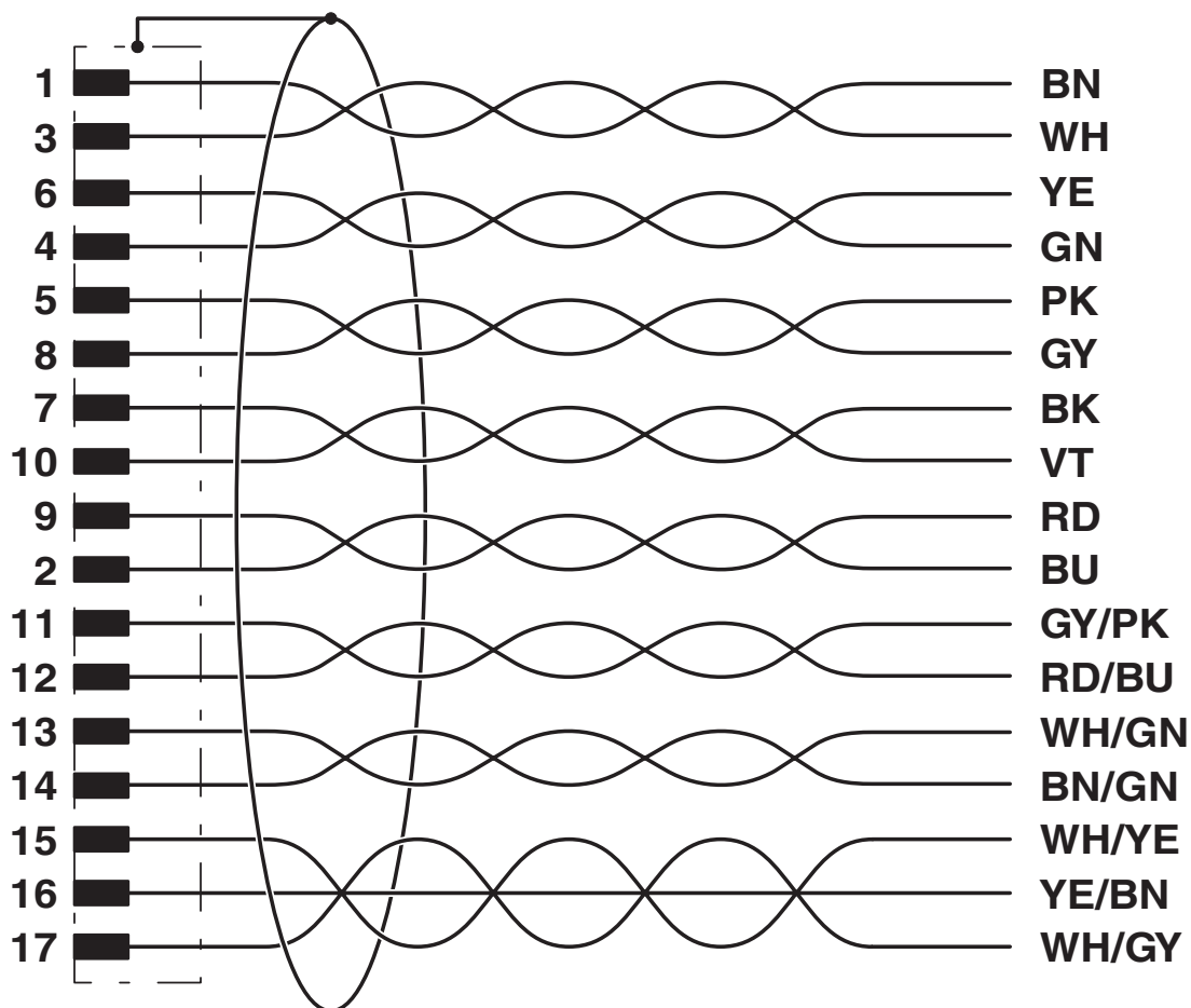
Kopplingsschema
