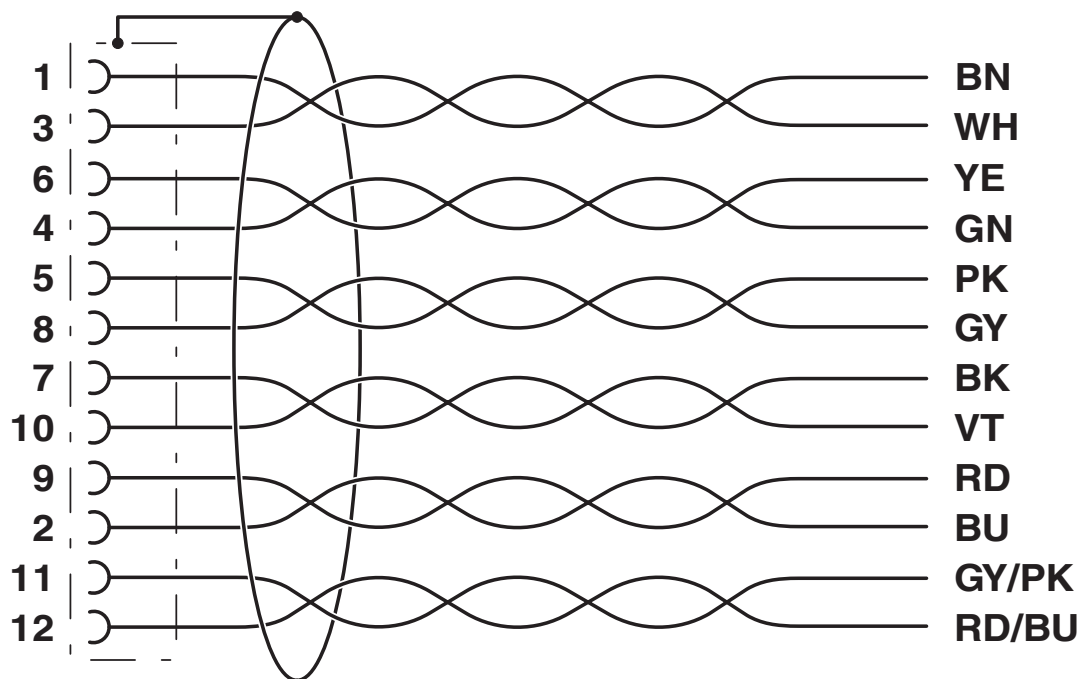
Kopplingsschema
