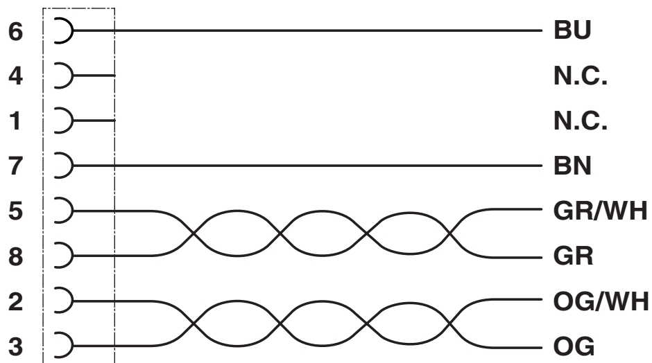
Kopplingsschema
