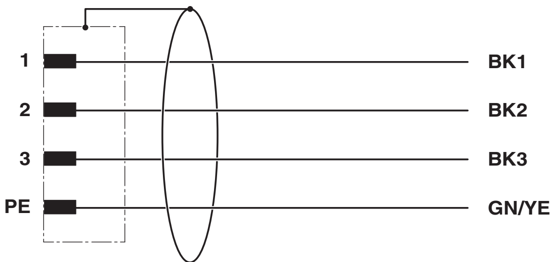
Kopplingsschema
