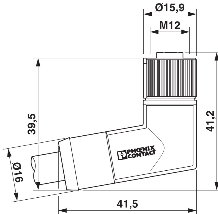
Måttskiss
