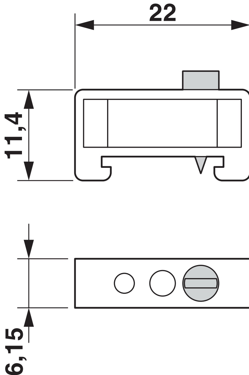
Måttskiss
