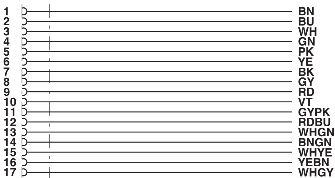
Anslutna M12-honkontakter
