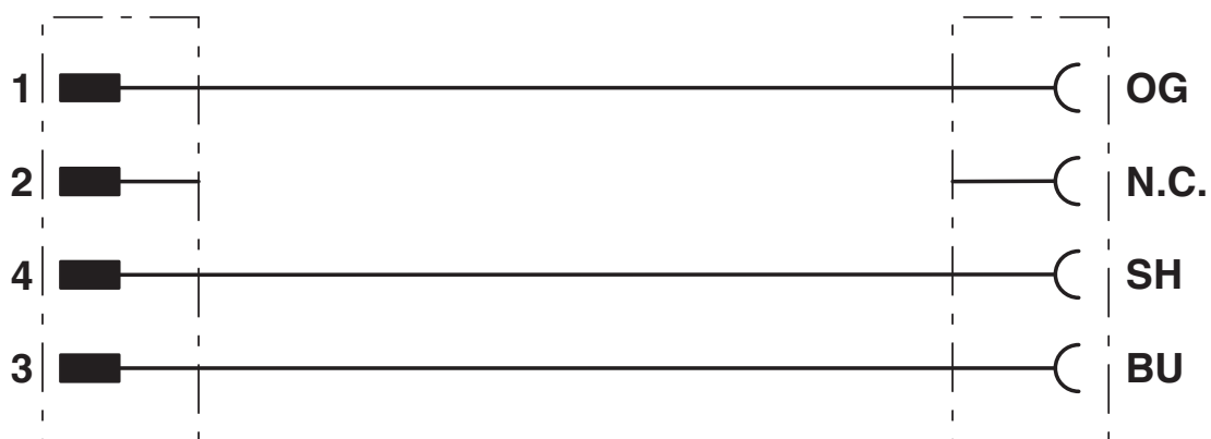
Kopplingsschema
