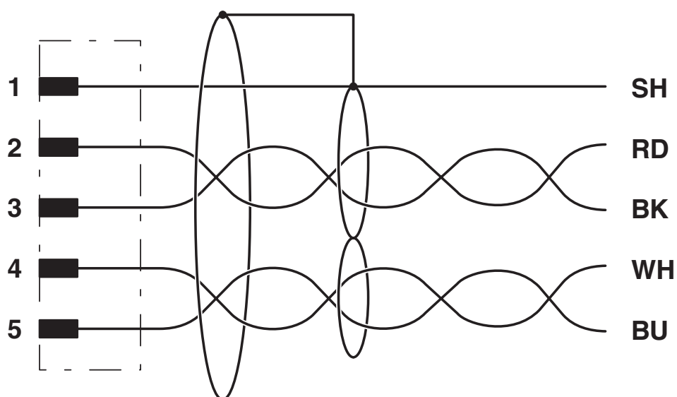
Kopplingsschema
