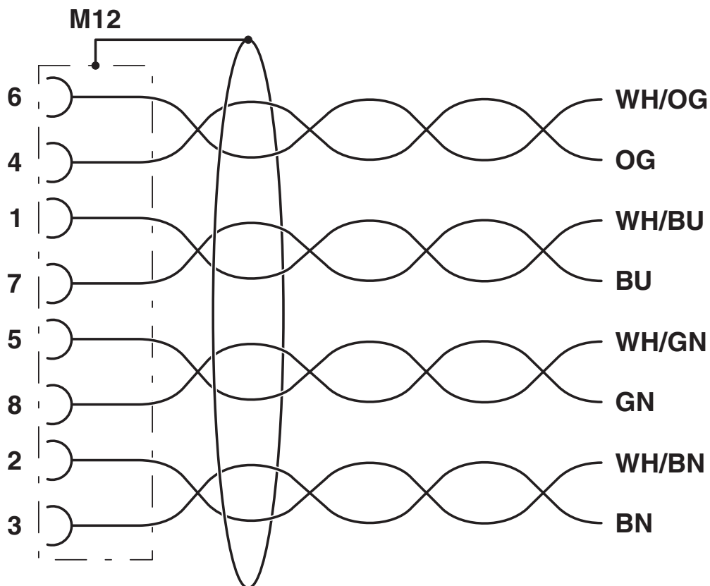
Kopplingsschema
