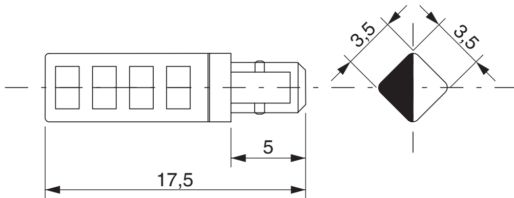
Måttskiss
