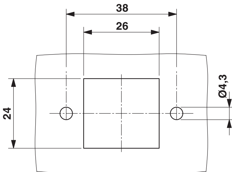
Måttskiss
