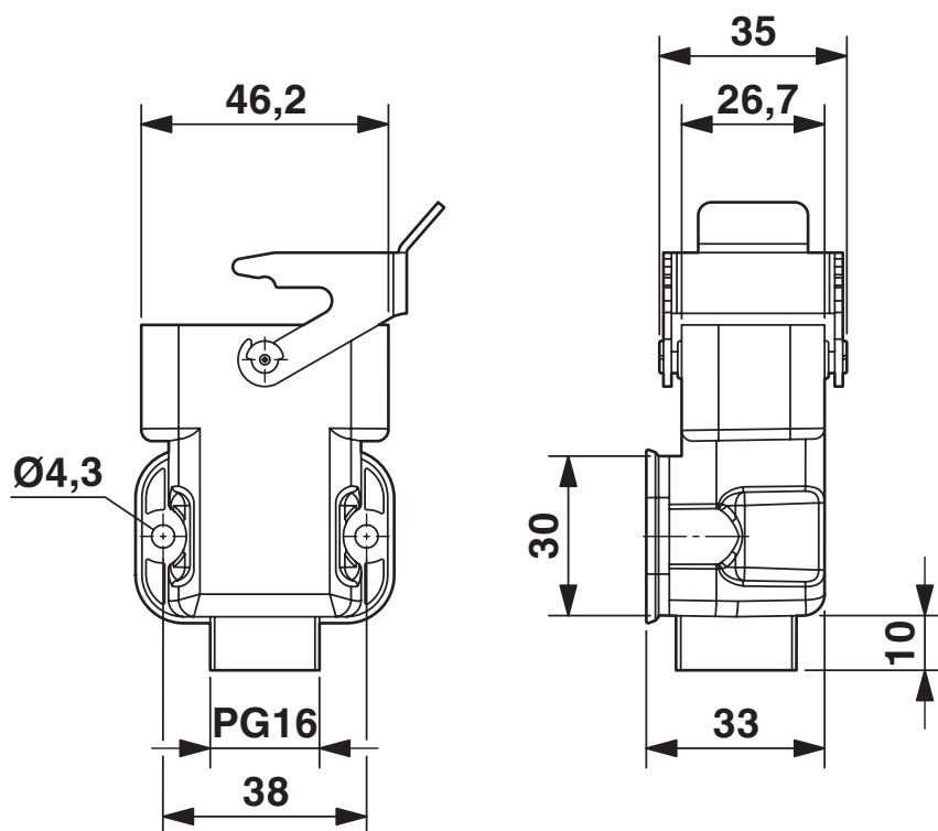
Måttskiss
