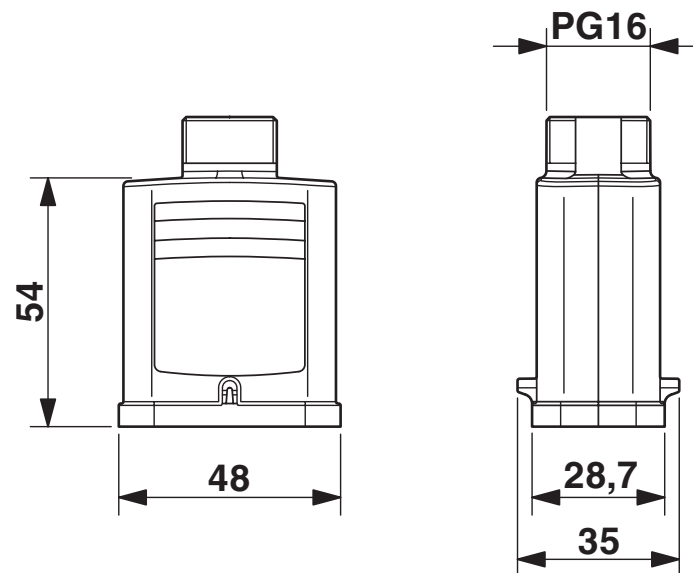
Måttskiss
