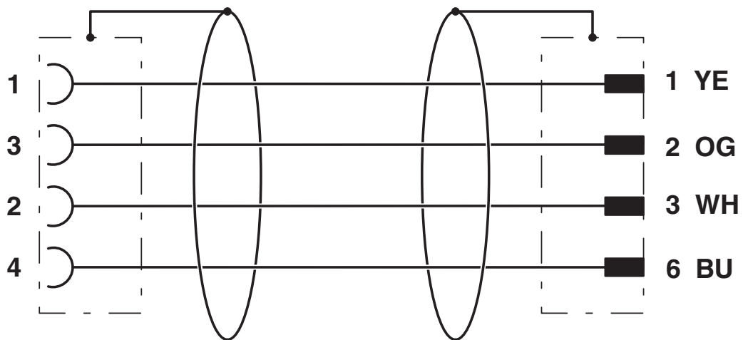
Kopplingsschema
