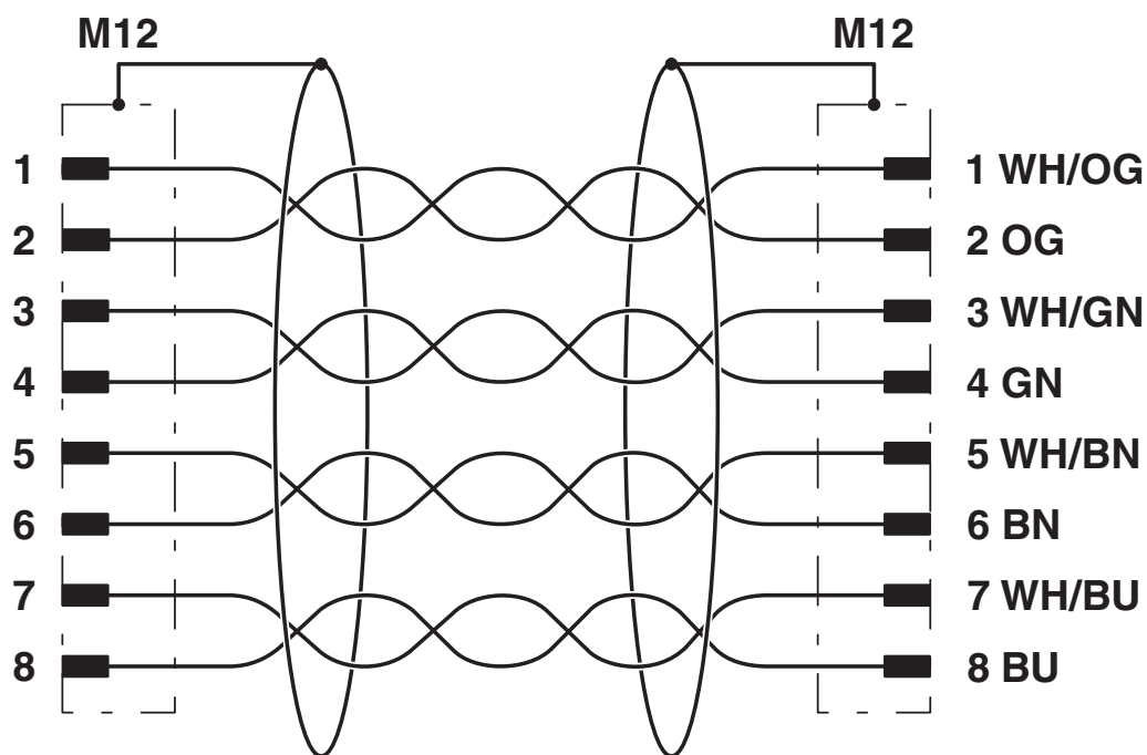
Kopplingsschema
