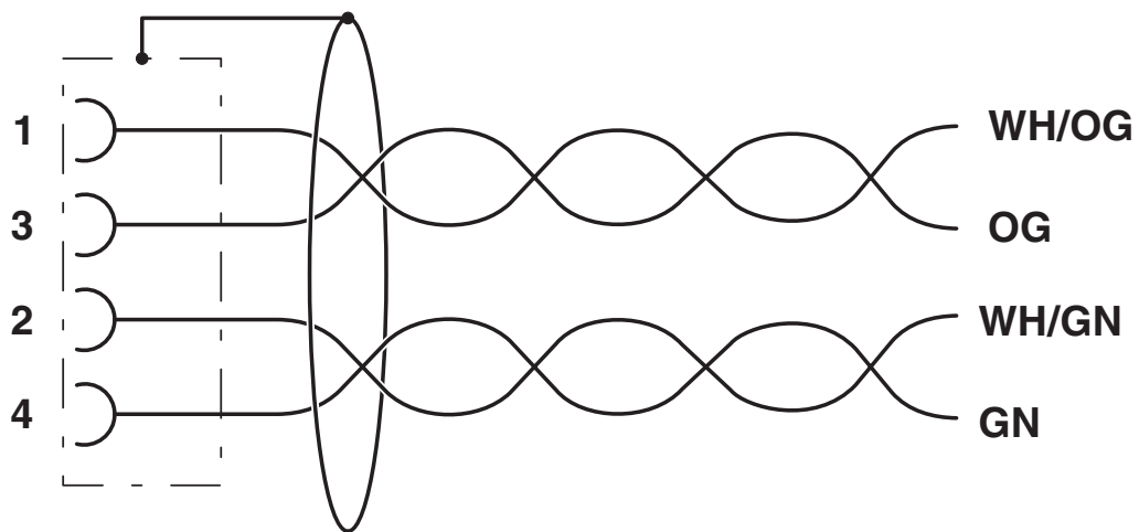
Kopplingsschema
