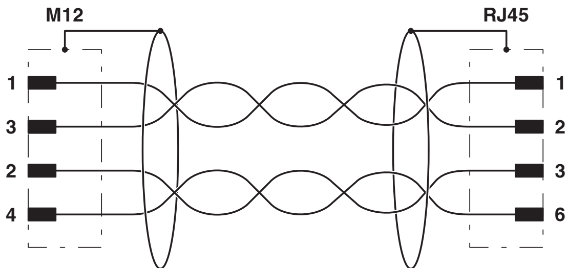
Kopplingsschema
