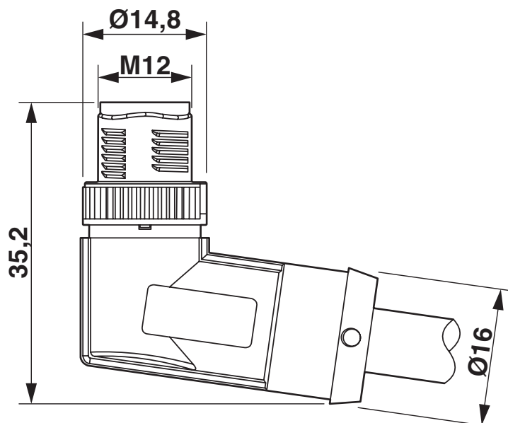
Måttskiss
