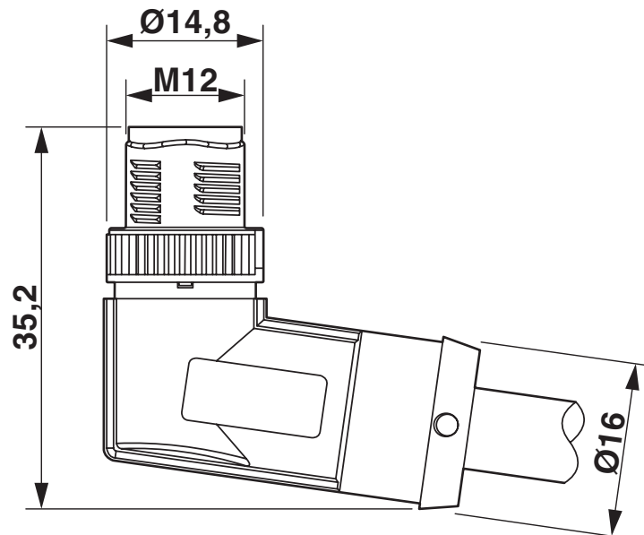
Måttskiss
