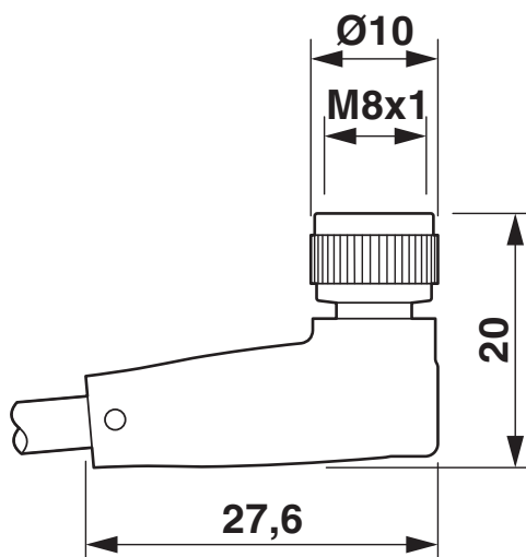
Måttskiss
