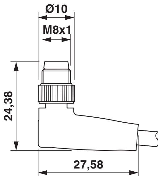
Måttskiss
