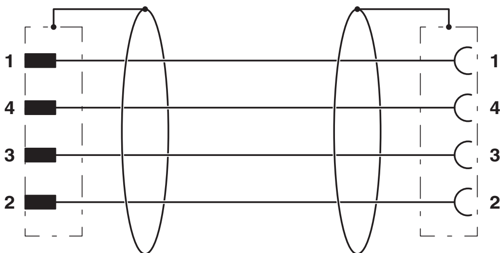
Kopplingsschema
